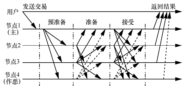
图 8 PBFT 协议示意
